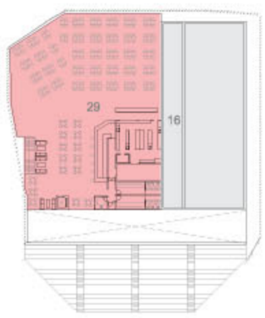
Planta 3 Esc: 1:500
